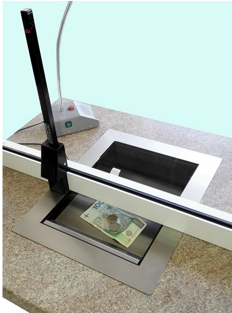
Jednoczęściowy moduł MZ4 klejony do szyby nad podajnikiem z przesuwaną łódką. W tle widoczna baza kasjera IB-IKG-D3
