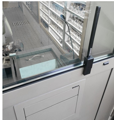
Interkom OPTIMUS zainstalowany na w witrynie kasowej z podajnikiem szufladowym (szufladą podawczą)
