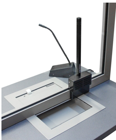
Interkom CONTACTA zainstalowany na oknie kasowym z blatem i podajnikiem w blacie
