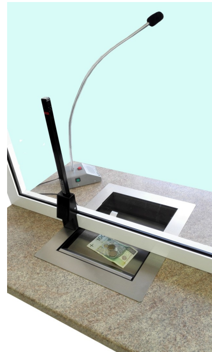
HIT !!! Zestaw uniwersalny optymalny: Moduł MZ4 mocowany do szyby + baza IB-IKG-D3
